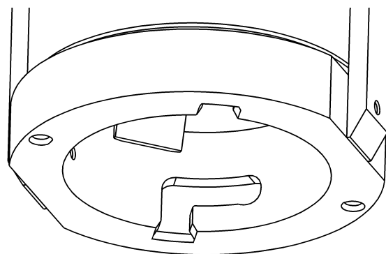
Obr. 3: Spodní část pláště transportního kontejneru
