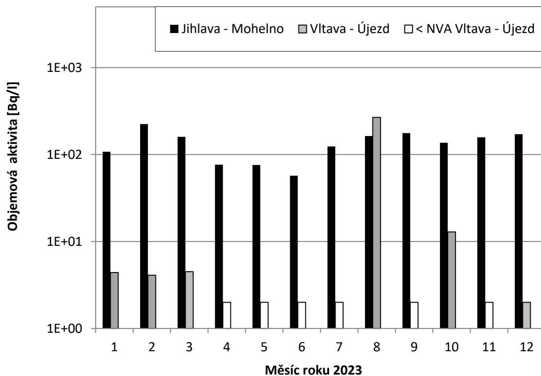
Obr. 21 Objemová aktivita ^3\text{H} v řece Jihlavě (profil Mohelno) a v řece Vltavě (profil Újezd) v roce 2022 (odběr a měření SÚRO České Budějovice)
