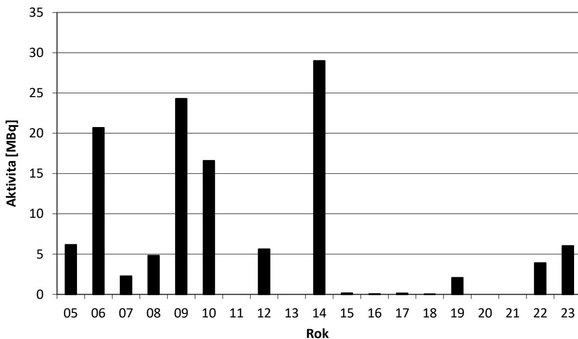
Obr. 15c Bilance kapalných výpustí radionuklidů emitujících záření beta z odběrů v čistící stanici ÚJV Řež v období 2005 až 2023 – celková aktivita beta přepočtená na referenční radionuklid ^{137}\text{Cs} (vzorkování a měření ÚJV Řež)
