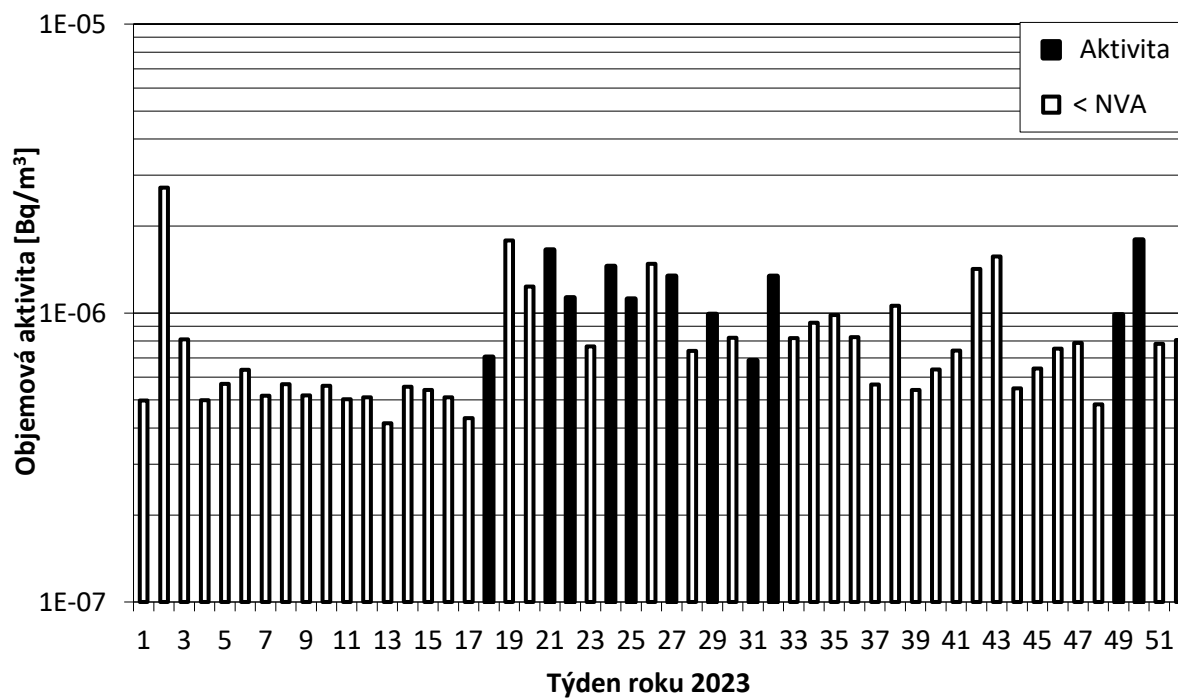
Obr. 7b Objemová aktivita ^{137}\text{Cs} v aerosolu v ovzduší v roce 2023 – OM Plzeň – Klatovská (vzorkování SÚRO České Budějovice – pracoviště Plzeň, měření SÚRO České Budějovice)
