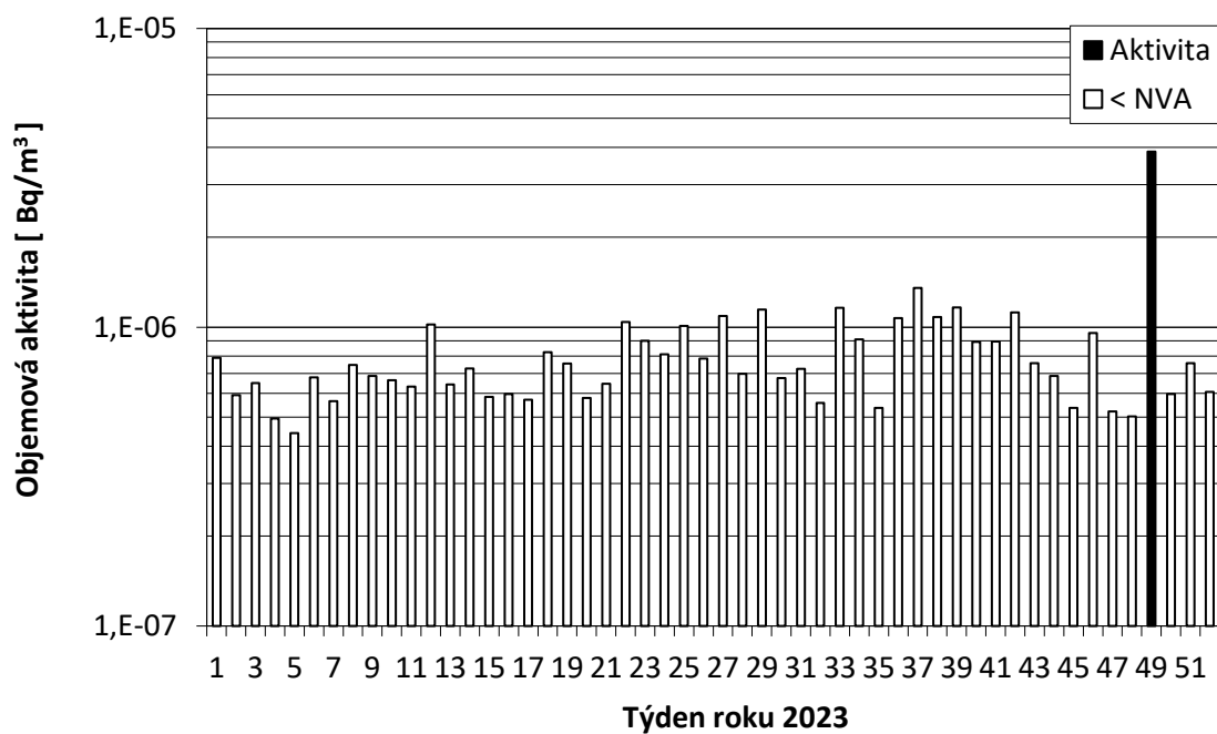
Obr. 17b Objemová aktivita ^{137}\text{Cs} ve vzdušném aerosolu v roce 2023 ve spojených vzorcích odebraných na stanicích radiční kontroly v okolí a v areálu JE Temelín (odběr a měření LRKO JE Temelín)
