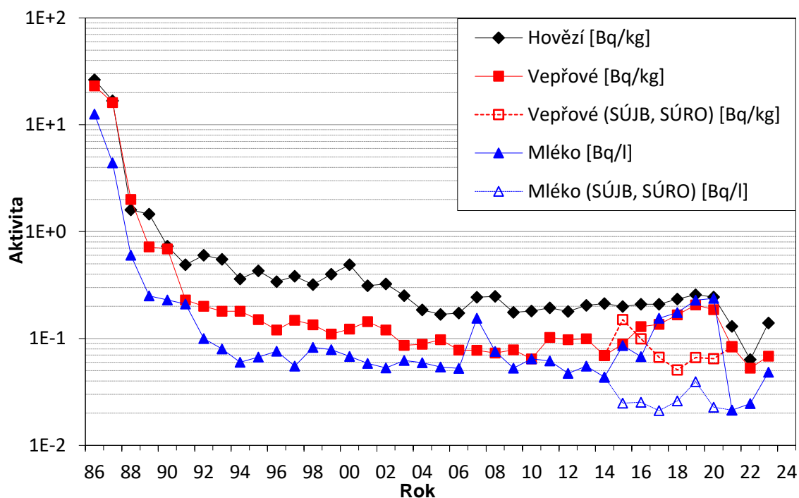
Obr. 13 Průměrné roční hmotnostní aktivity ^{137}\text{Cs} ve vepřovém a hovězím masu a objemové aktivity ^{137}\text{Cs} v mléce od roku 1986 (vzorkování a měření RC SÚJB, SÚRO a od roku 2004 i SVÚ)
