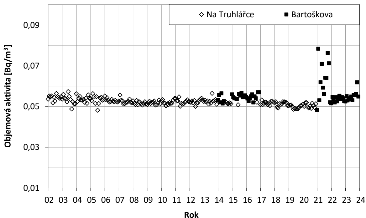
Obr. 9a Objemová aktivita ^{14}\text{C} v ovzduší ve formě \text{CO}_2 , měsíční hodnoty – OM Praha (do 2013 vzorkování a měření ODZ ÚJF AV, od 2014 do roku 2017 také SÚRO Praha, od roku 2021 pouze SÚRO Praha)
