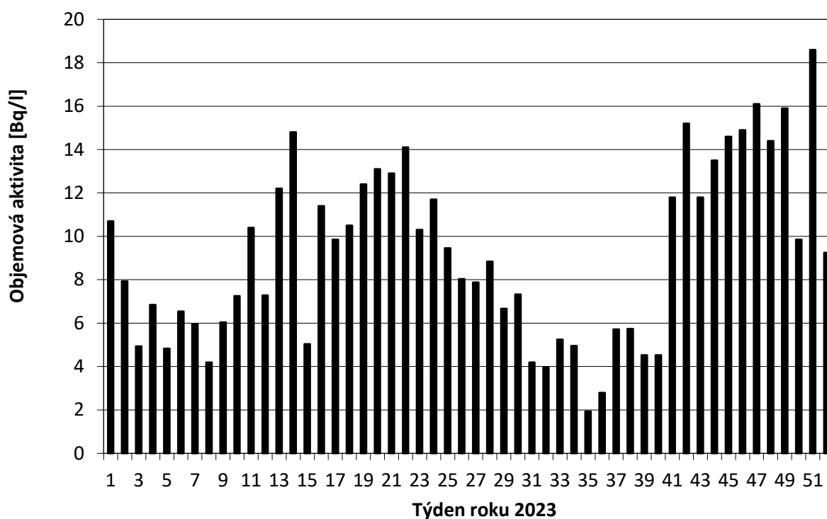
Obr. 12c Objemová aktivita ^3\text{H} v povrchové vodě v roce 2023 – povodí Vltava – profil Praha-Podolí (Vltava), (vzorkování a měření VÚV TGM Praha)
