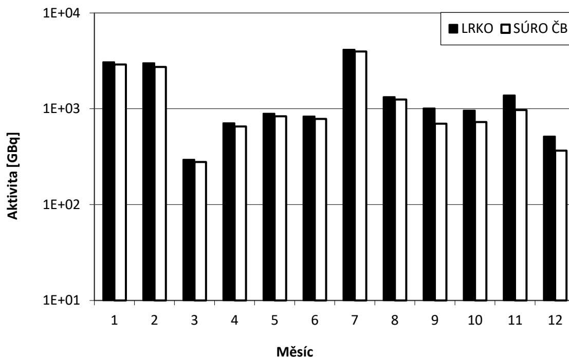
Obr. 19b Objemová aktivita ^3\text{H} v odpadním kanále JE Dukovany v roce 2023 (porovnání hodnot naměřených SÚRO a LRKO provozovatele, odběr JE Dukovany, měření SÚRO České Budějovice a LRKO JE Dukovany)
