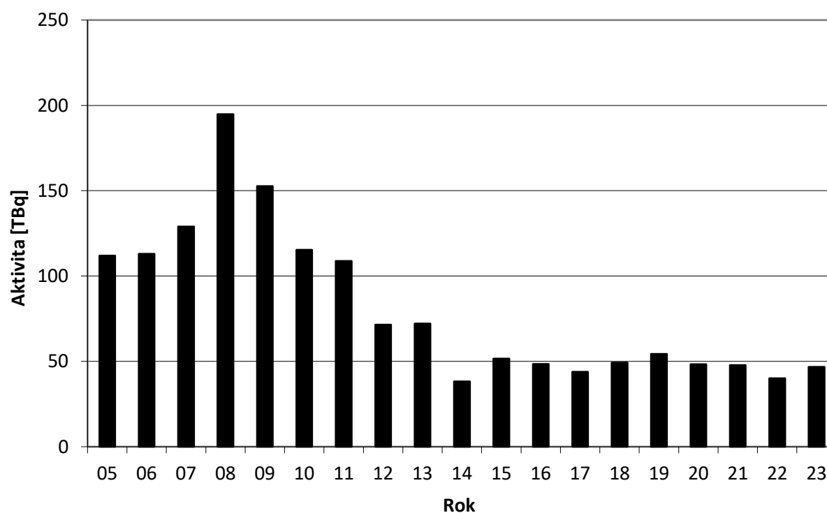
Obr. 15a Bilance plyných výpustí – vzácné plyny ( ^{41}\text{Ar} ) z odběrů ve ventilačním komínu ÚJV Řež v období 2005 – 2023 (vzorkování a měření ÚJV Řež)
