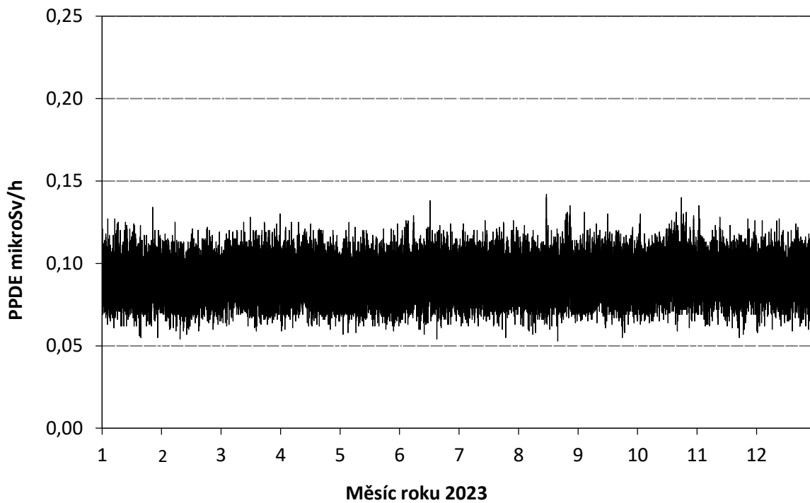
Obr. 2a Příkon prostorového dávkového ekvivalentu (PPDE) – SVZ SÚJB Praha (měřicí místo resort SÚJB)
