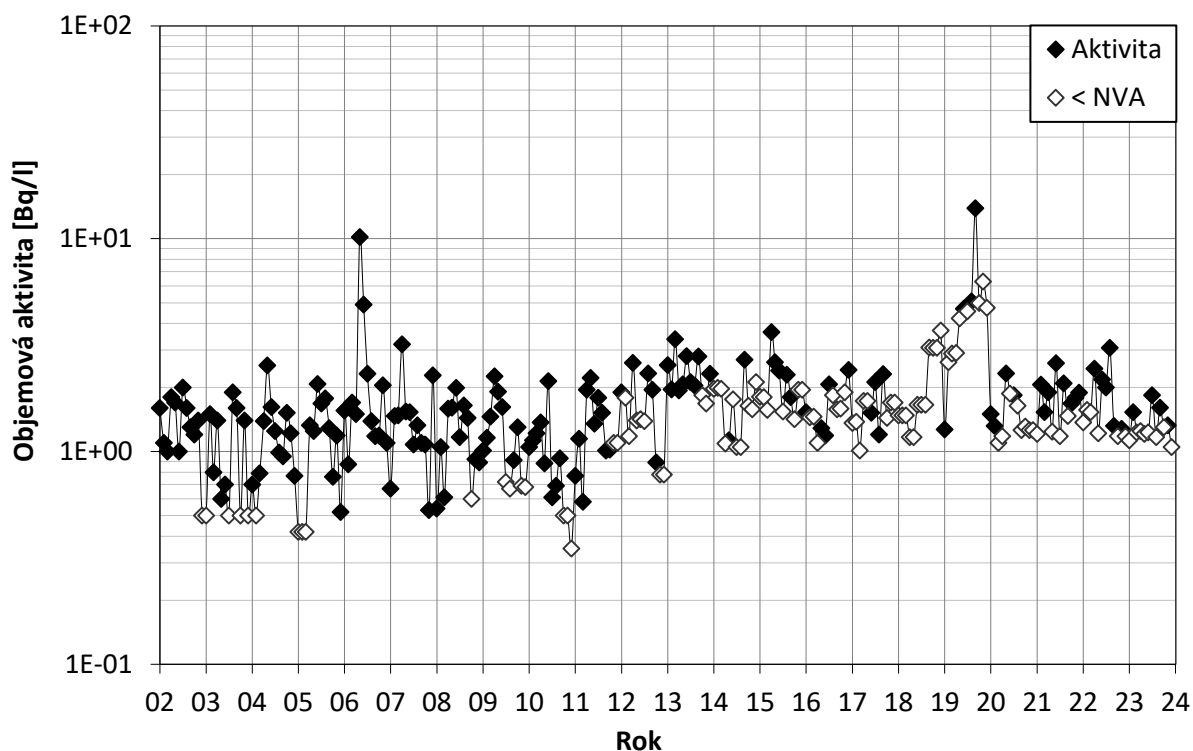
Obr. 11b Objemová aktivita 3 H ve srážkách od roku 2003, měsíční hodnoty – OM Praha (vzorkování a měření SÚRO Praha)
