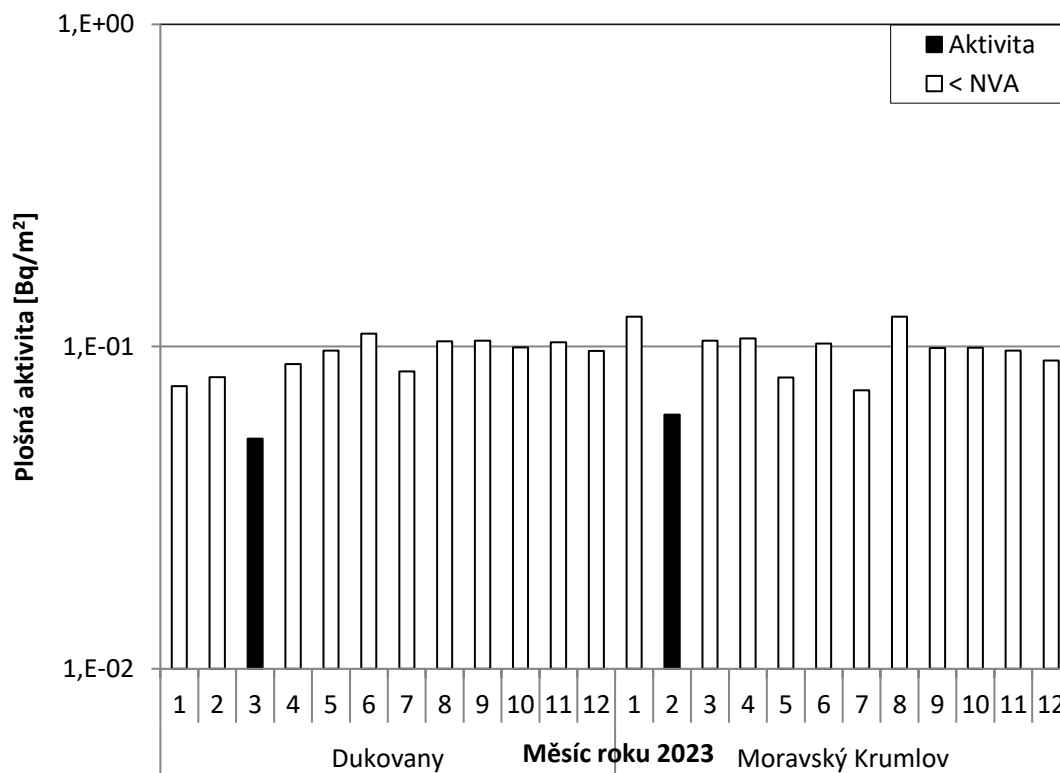
Obr. 22a Plošná aktivita ^{137}\text{Cs} ve spadech v okolí JE Dukovany v roce 2023 (měsíční hodnoty; odběr a měření SÚRO České Budějovice)
