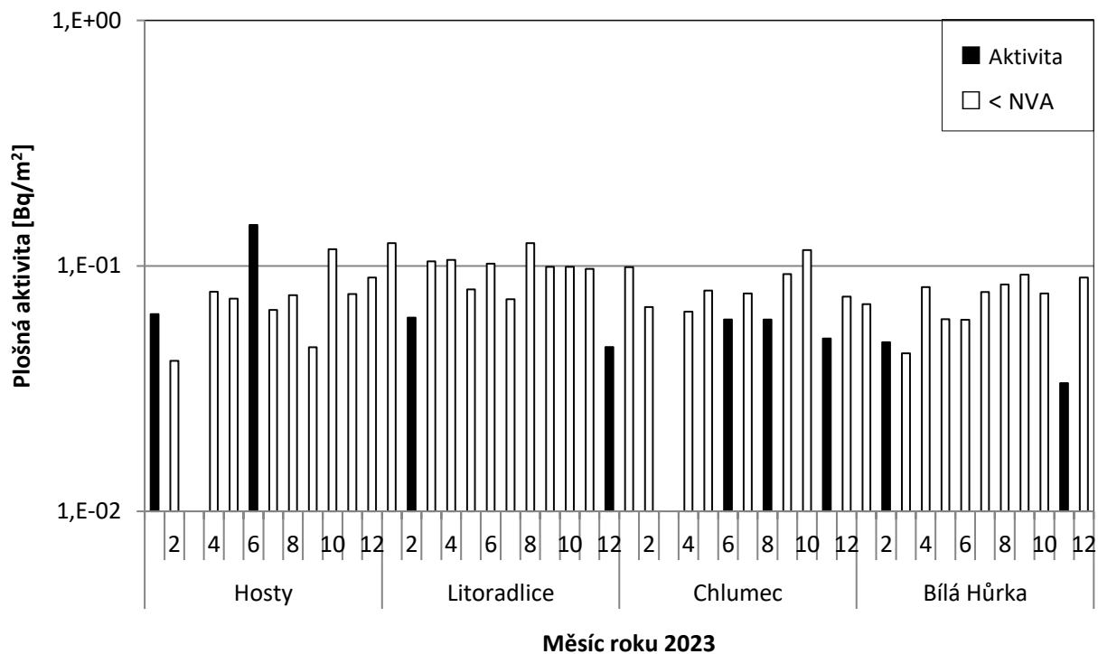
Obr. 22b Plošná aktivita 137 Cs ve spadech v okolí JE Temelín v roce 2023 (měsíční hodnoty v jednotlivých lokalitách; odběr a měření SÚRO České Budějovice)
