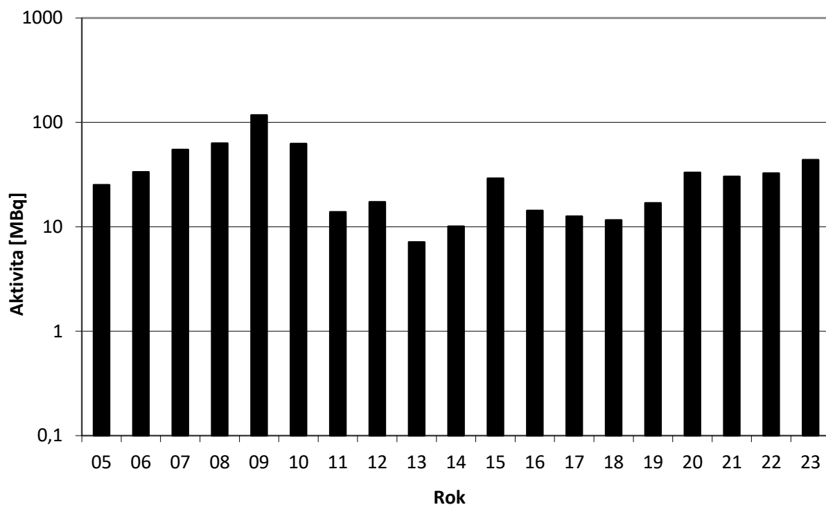
Obr. 15c Bilance kapalných výpustí radionuklidů emitujících záření beta z odběrů v čistící stanici ÚJV Řež v období 2005 až 2023 – celková aktivita beta přepočtená na referenční radionuklid ^{137}\text{Cs} (vzorkování a měření ÚJV Řež)
