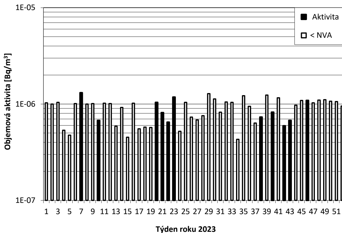
Obr. 7a Objemová aktivita ^{137}\text{Cs} v aerosolu v ovzduší v roce 2023 – OM Hradec Králové – Piletice (vzorkování a měření SÚRO Hradec Králové)
