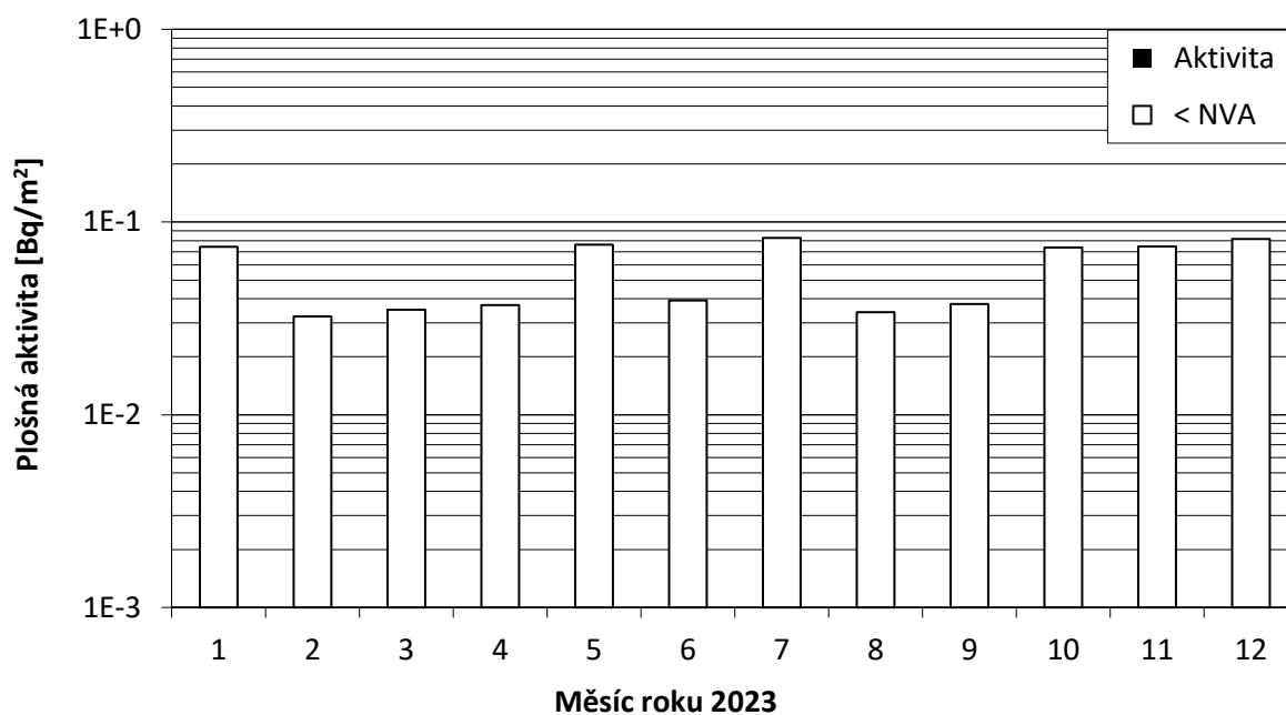
Obr. 10a Plošná aktivita ^{137}\text{Cs} ve spadech v roce 2023, měsíční hodnoty – OM Ústí nad Labem - Habrovce (vzorkování SÚRO Praha, měření SÚRO Hradec Králové)
