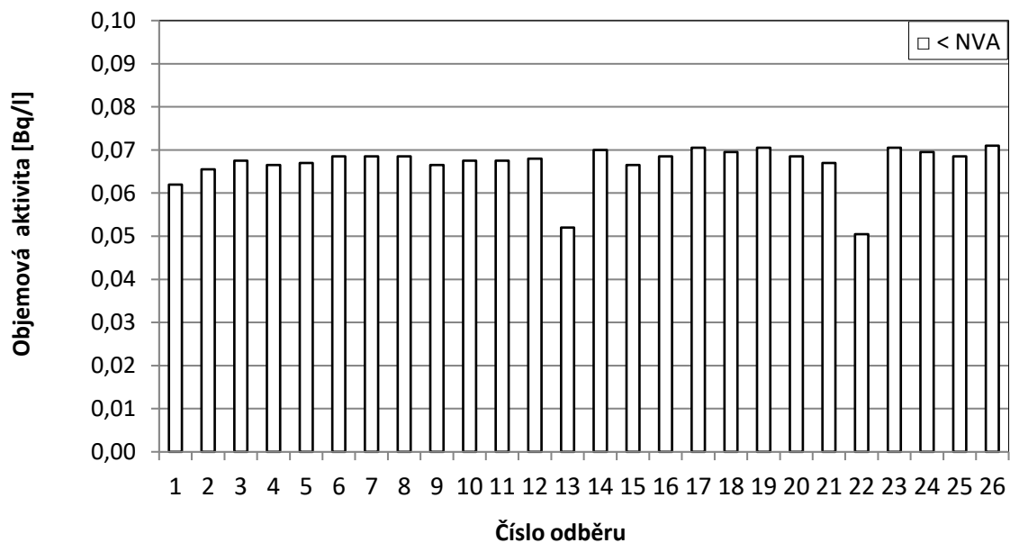
Obr. 18b Objemová aktivita ^{137}\text{Cs} v mléce v roce 2023 ve vzorcích odebraných v kravínech v ZHP JE Temelín (odebírání se jednou za 14 dní; odběr a měření LRKO JE Temelín)
