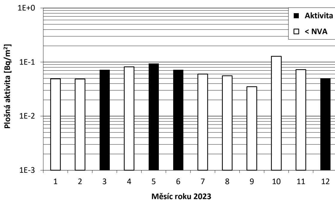
Obr. 10b Plošná aktivita ^{137}\text{Cs} ve spadech v roce 2023, měsíční hodnoty – OM České Budějovice – U nemocnice (vzorkování a měření SÚRO České Budějovice)
