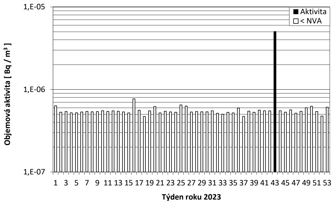
Obr. 17a Objemová aktivita ^{137}\text{Cs} ve vzdušném aerosolu v roce 2023 ve spojených vzorcích odebraných na odběrových místech v okolí a v areálu JE Dukovany (odběr a měření LRKO JE Dukovany)
