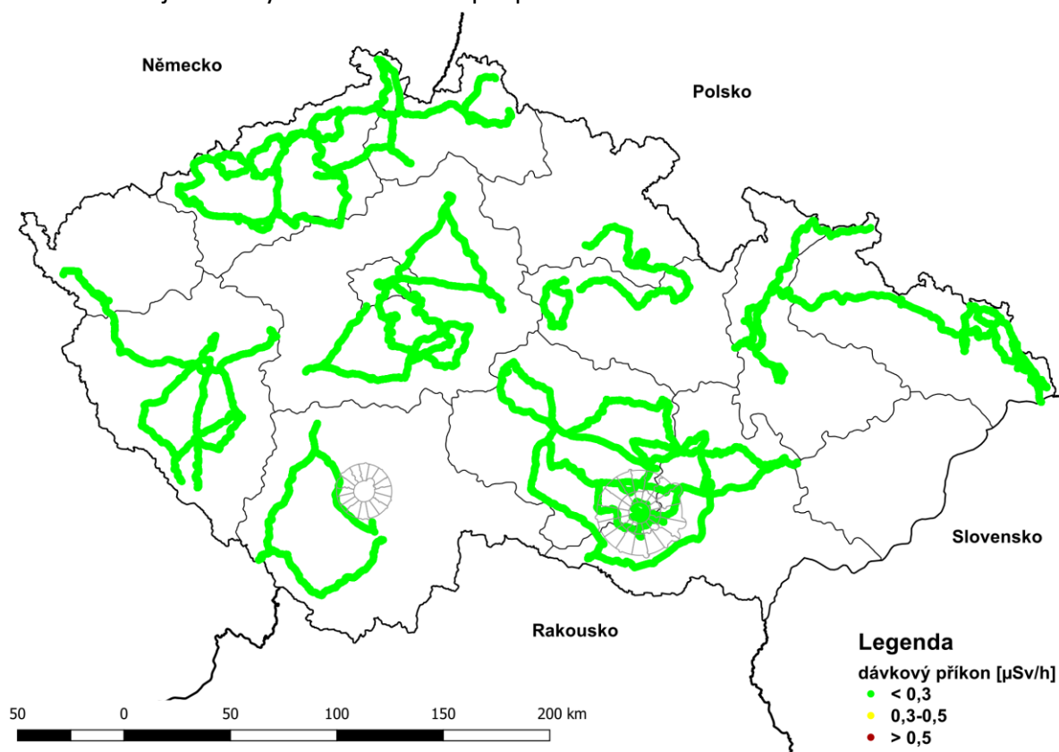
Obr. 4 Měření příkonů prostorového dávkového ekvivalentu po trasách pojezdu jednotlivých mobilních skupin při svozu a rozvozu TLD v lednu roku 2024
