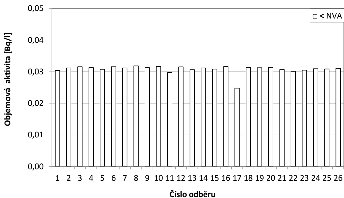
Obr. 18a Objemová aktivita ^{137}\text{Cs} v mléce v roce 2024 ve vzorcích odebraných v kravínech v ZHP JE Dukovany (odebírání se jednou za 14 dní; odběr a měření LRKO JE Dukovany)
