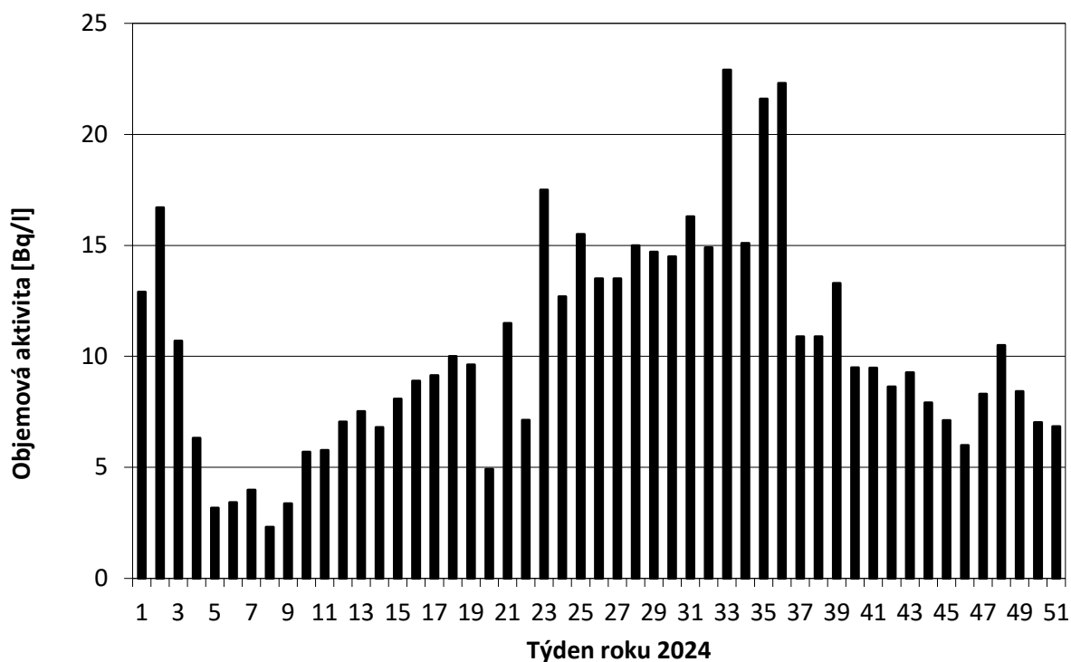
Obr. 12c Objemová aktivita ^3\text{H} v povrchové vodě v roce 2024 – povodí Vltava – profil Praha-Podolí (Vltava), (vzorkování a měření VÚV TGM Praha)
