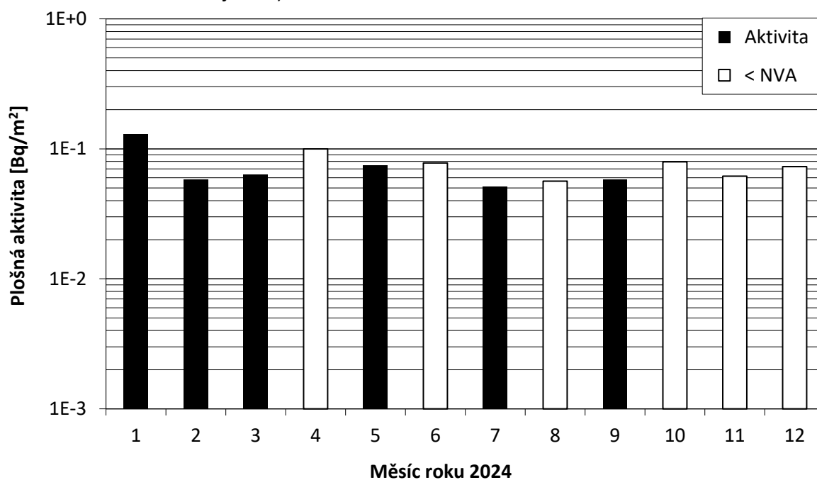
Obr. 10b Plošná aktivita ^{137}\text{Cs} ve spadech v roce 2024, měsíční hodnoty – OM Plzeň – Klatovská (vzorkování SÚRO České Budějovice – pracoviště Plzeň, měření SÚRO České Budějovice)
