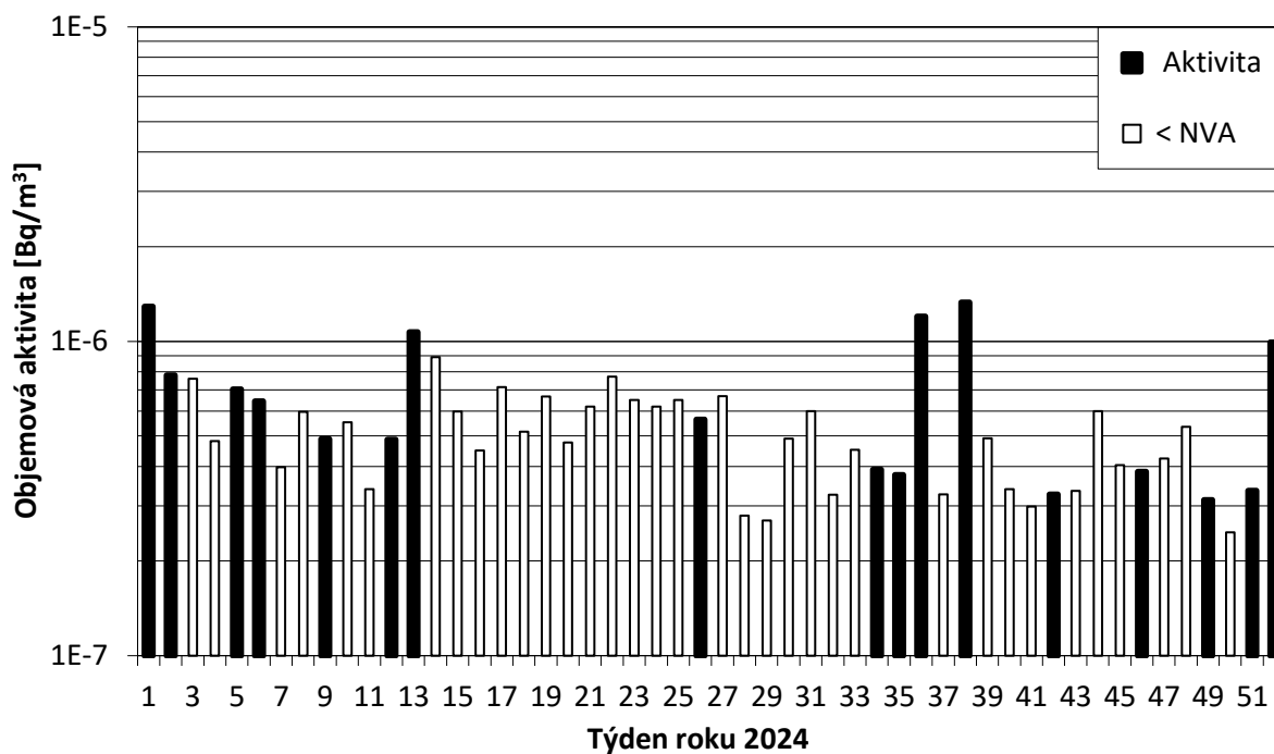
Obr. 7b Objemová aktivita ^{137}\text{Cs} v aerosolu v ovzduší v roce 2024 – OM Brno - Arboretum (vzorkování SÚRO České Budějovice – pracoviště Brno, měření SÚRO České Budějovice)
