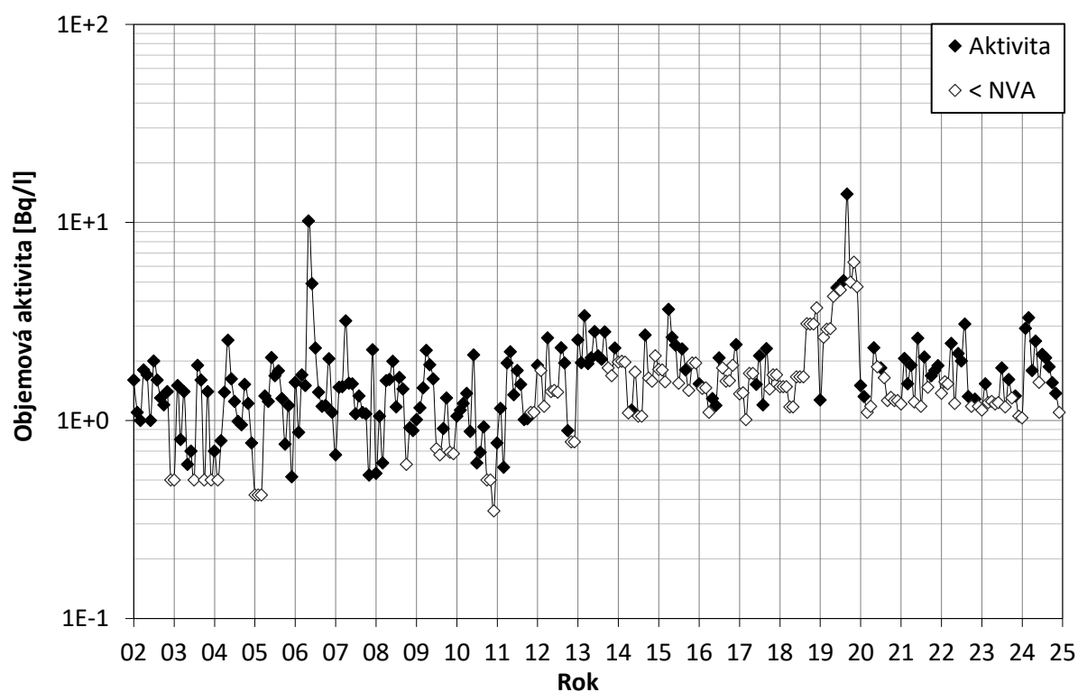
Obr. 11b Objemová aktivita ^3\text{H} ve srážkách od roku 2002, měsíční hodnoty – OM Praha (vzorkování a měření SÚRO Praha)
