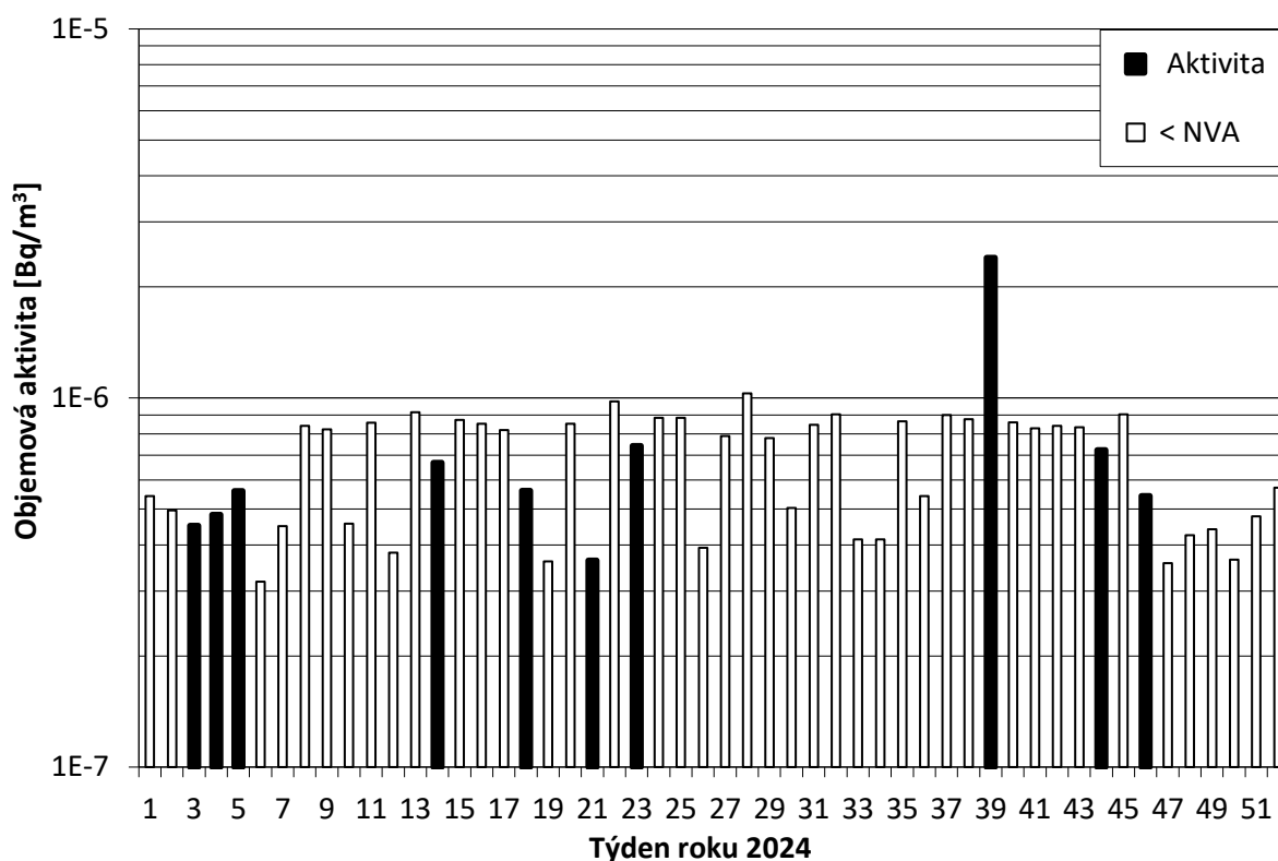
Obr. 7a Objemová aktivita ^{137}\text{Cs} v aerosolu v ovzduší v roce 2024 – OM Ústí nad Labem - Habrovice (vzorkování SÚRO Praha, měření SÚRO Hradec Králové)
