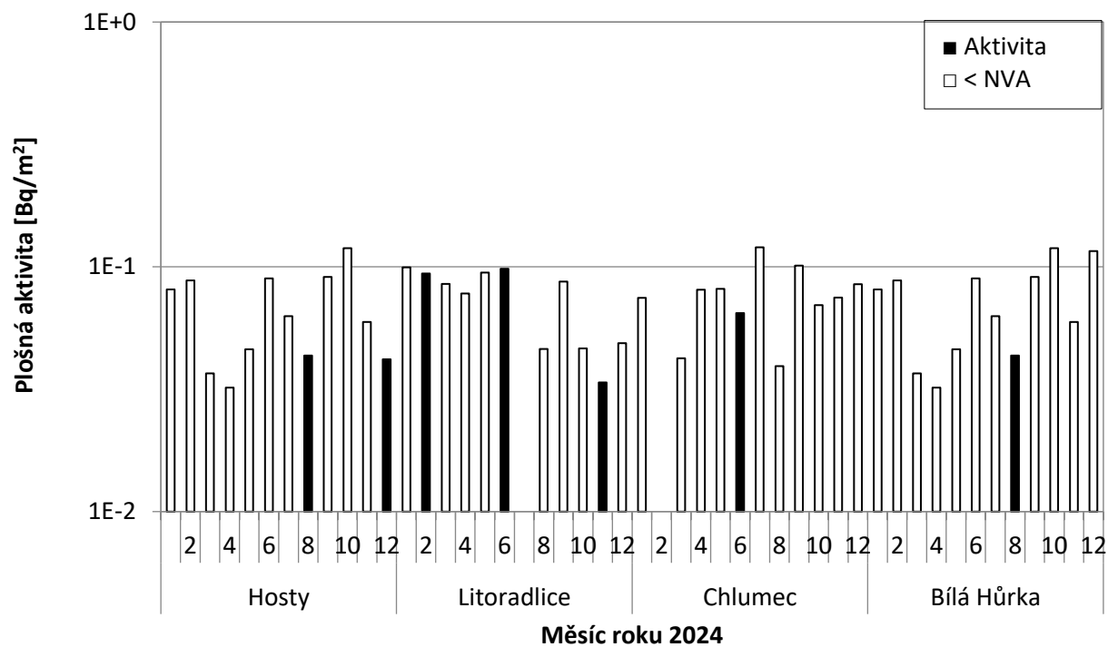
Obr. 22b Plošná aktivita ^{137}\text{Cs} ve spadech v okolí JE Temelín v roce 2024 (měsíční hodnoty v jednotlivých lokalitách; odběr a měření SÚRO České Budějovice)
