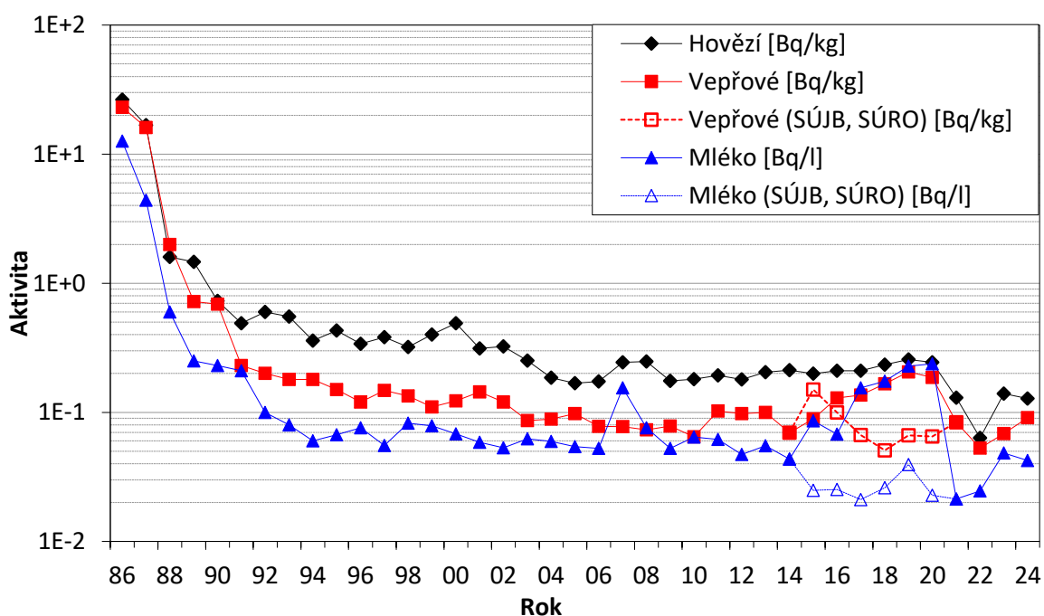
Obr. 13 Průměrné roční hmotnostní aktivity ^{137}\text{Cs} ve vepřovém a hovězím masu a objemové aktivity ^{137}\text{Cs} v mléce od roku 1986 (vzorkování a měření RC SÚJB, SÚRO a od roku 2004 i SVÚ)
