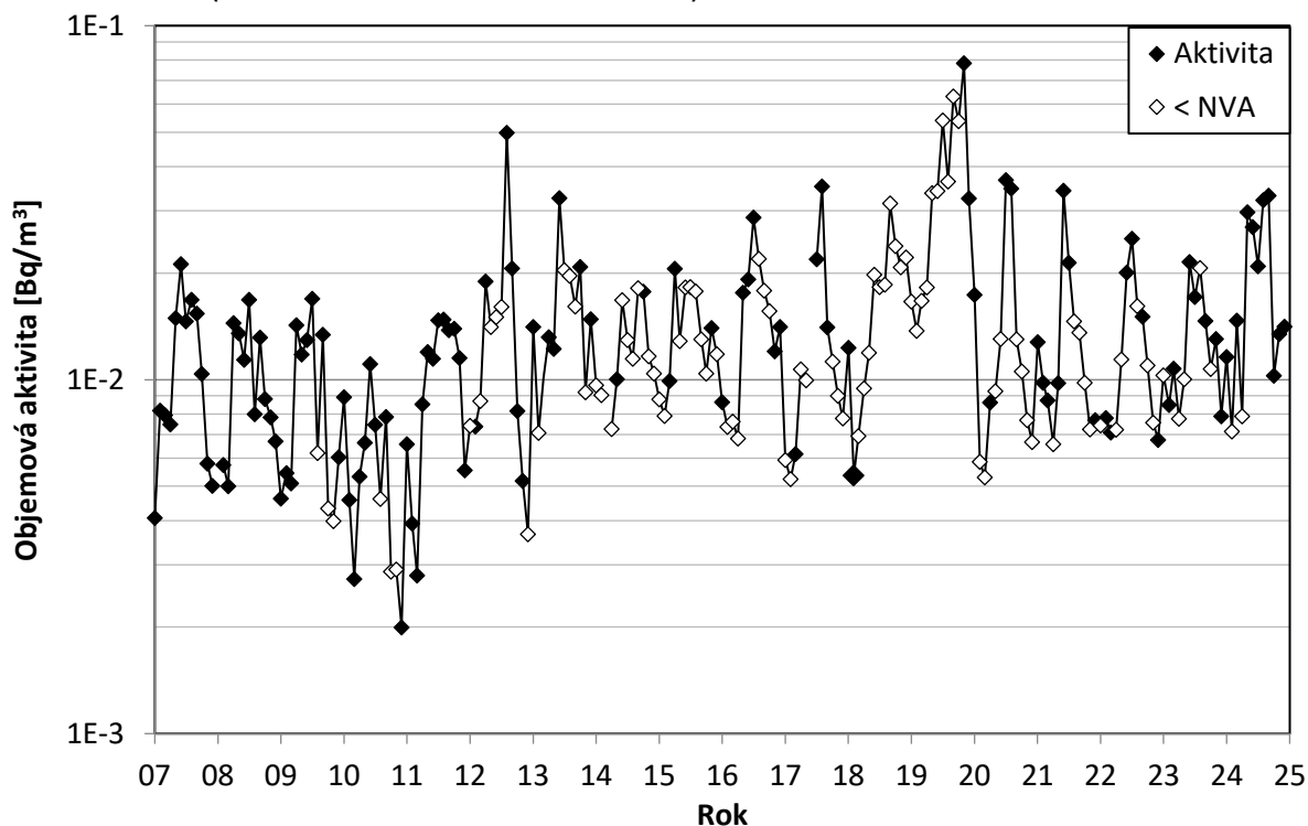
Obr. 9b Objemová aktivita ^3\text{H} ve formě HTO v ovzduší, měsíční hodnoty – OM Praha (vzorkování a měření SÚRO Praha)
