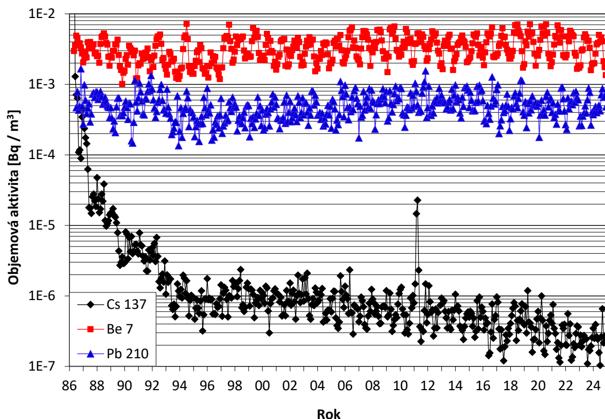
Obr. 8a Objemová aktivita vybraných radionuklidů v aerosolu v ovzduší, měsíční průměry od roku 1986 – OM Praha (vzorkování a měření SÚRO Praha)
