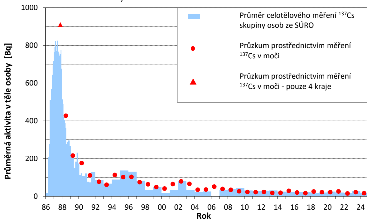
Obr. 14 Vývoj retence ^{137}\text{Cs} u českého obyvatelstva po černobylské havárii (vzorkování a měření SÚRO)
