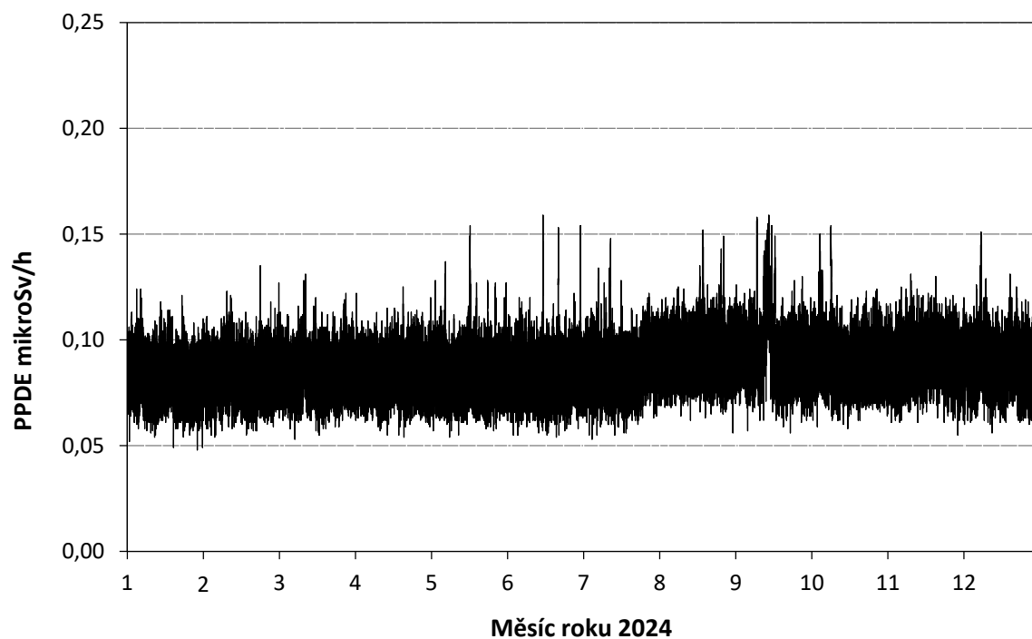
Obr. 16e Příkon prostorového dávkového ekvivalentu (PPDE) – SVZ Dukovany (měřicí místo ČHMÚ)
