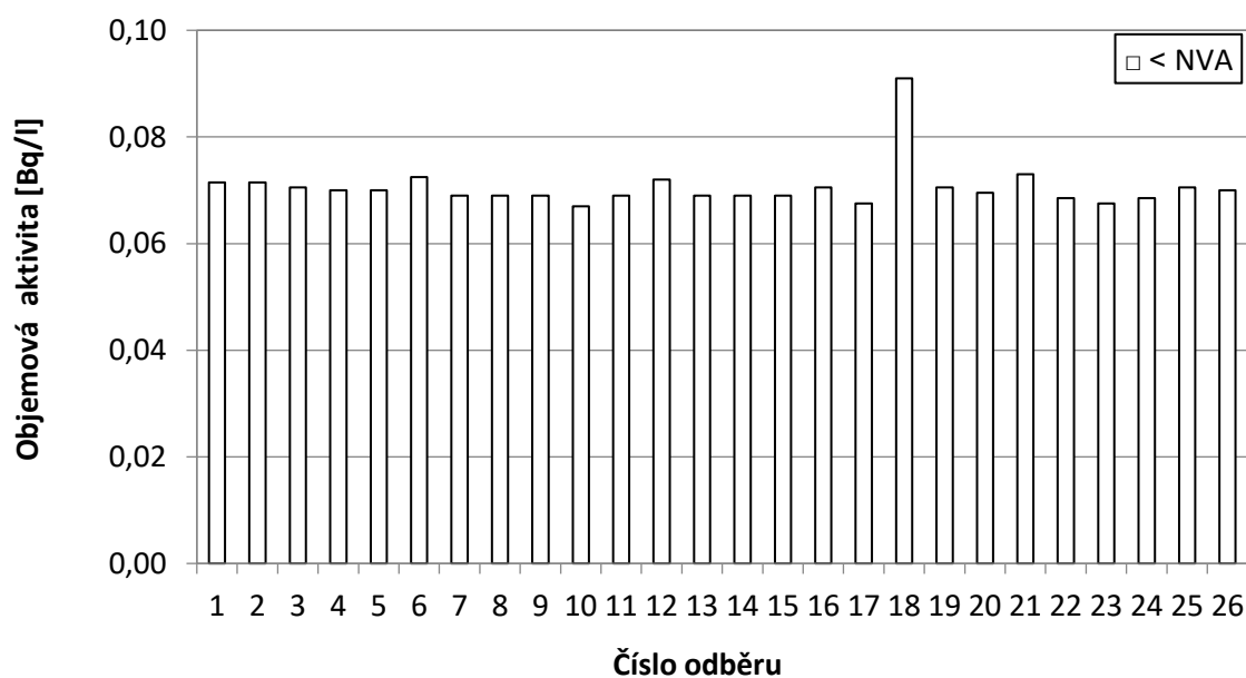
Obr. 18b Objemová aktivita ^{137}\text{Cs} v mléce v roce 2024 ve vzorcích odebraných v kravínech v ZHP JE Temelín (odebírání se jednou za 14 dní; odběr a měření LRKO JE Temelín)
