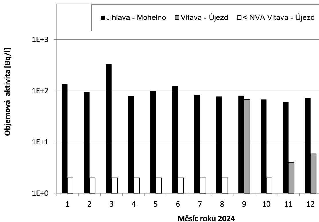
Obr. 21 Objemová aktivita ^3\text{H} v řece Jihlavě (profil Mohelno) a v řece Vltavě (profil Újezd) v roce 2024 (odběr a měření SÚRO České Budějovice)
