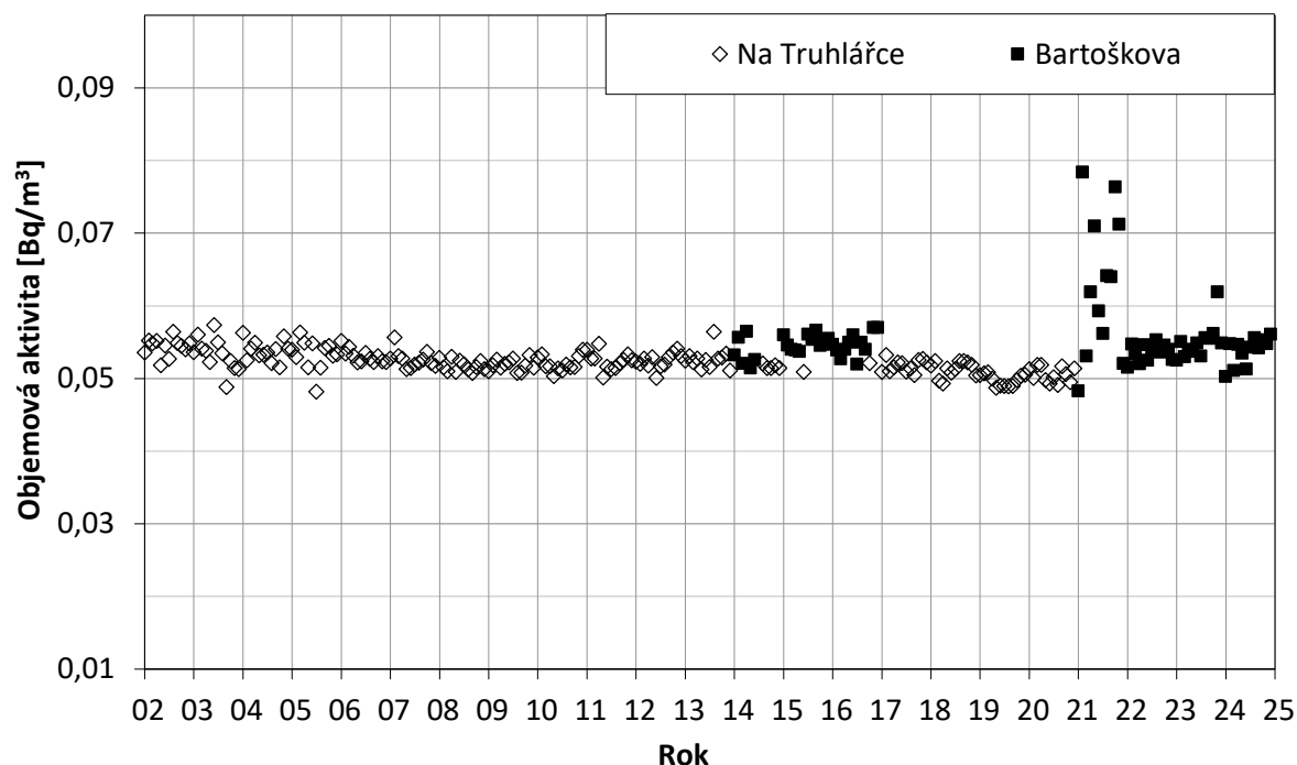
Obr. 9a Objemová aktivita ^{14}\text{C} v ovzduší ve formě \text{CO}_2 , měsíční hodnoty – OM Praha (do 2013 vzorkování a měření ODZ ÚJF AV, od 2014 do roku 2017 také SÚRO Praha, od roku 2021 pouze SÚRO Praha)
