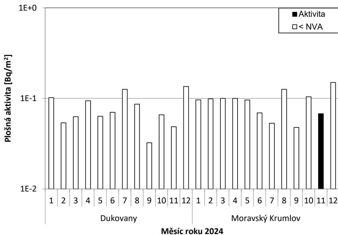
Obr. 22a Plošná aktivita ^{137}\text{Cs} ve spadech v okolí JE Dukovany v roce 2024 (měsíční hodnoty; odběr a měření SÚRO České Budějovice)
