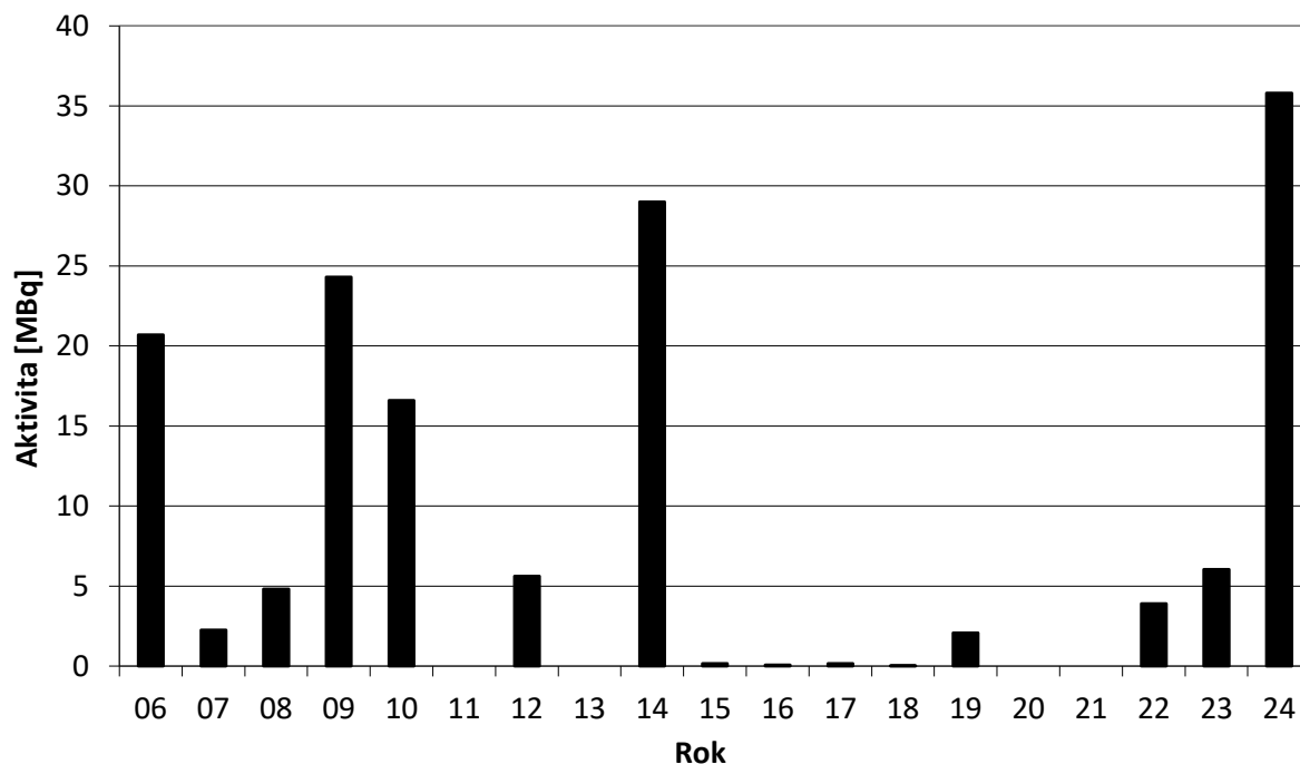
Obr. 15c Balance kapalných výpustí radionuklidů emitujících záření beta z odběrů v čistící stanici ÚJV Řež v období 2006 až 2024 – celková aktivita beta přepočtená na referenční radionuklid ^{137}\text{Cs} (vzorkování a měření ÚJV Řež)
