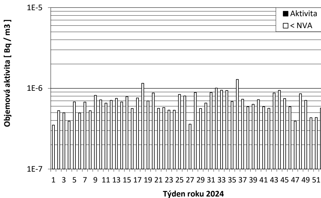
Obr. 17b Objemová aktivita ^{137}\text{Cs} ve vzdušném aerosolu v roce 2024 ve spojených vzorcích odebraných na stanicích radiální kontroly v okolí a v areálu JE Temelín (odběr a měření LRKO JE Temelín)
