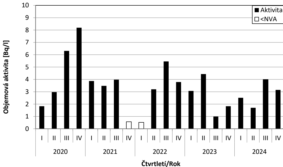
Obr. 12b Objemová aktivita ^3\text{H} v povrchové vodě za posledních 5let – povodí Morava – profil Lanžhot (Morava), (odběrové místo je Moravský Svatý Ján; vzorkování Povodí, s. p., měření VÚV TGM Praha)
