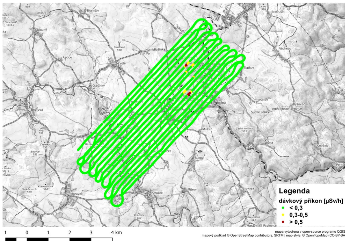
Obr. 5 Výsledky leteckého monitorování SÚRO a AČR
