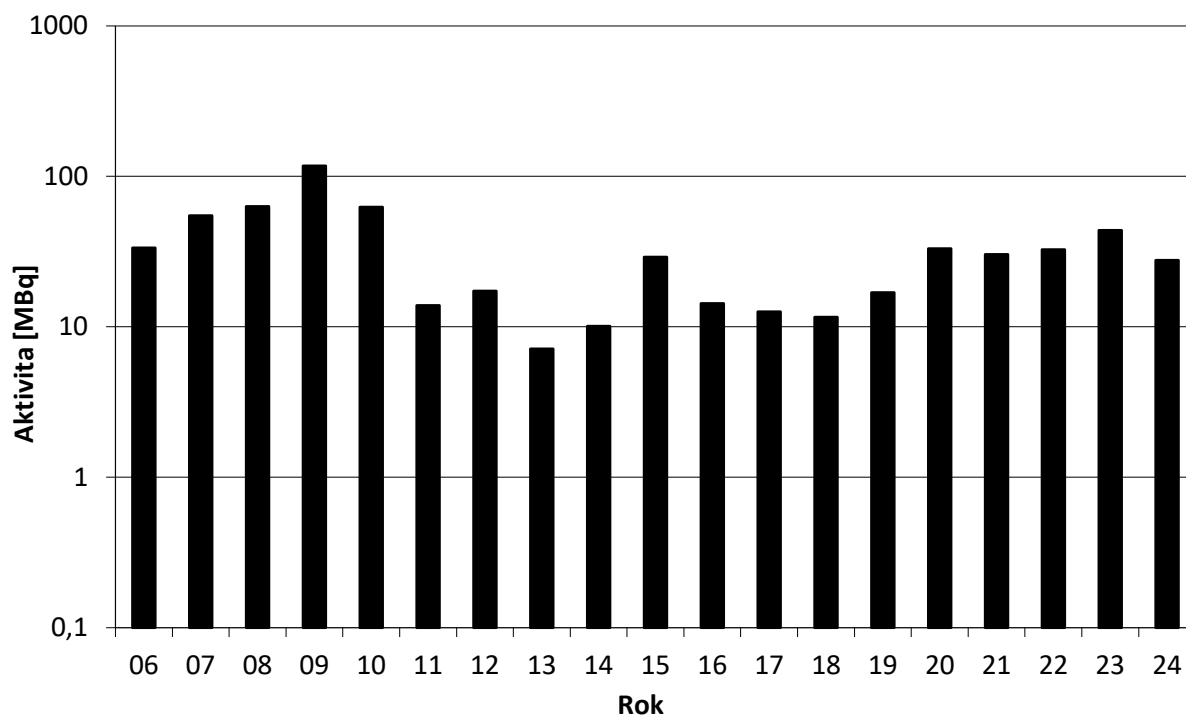
Obr. 15b Balance plyných výpustí – ^{131}\text{I} z odběrů ve ventilačním komínu ÚJV Řež v období 2006 – 2024 (vzorkování a měření ÚJV Řež)
