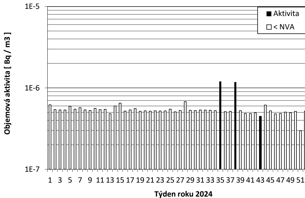
Obr. 17a Objemová aktivita ^{137}\text{Cs} ve vzdušném aerosolu v roce 2024 ve spojených vzorcích odebraných na odběrových místech v okolí a v areálu JE Dukovany (odběr a měření LRKO JE Dukovany)
