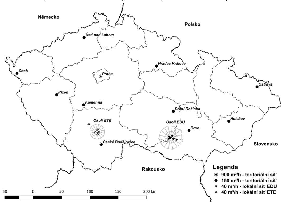
Obr. 6 Mapa rozmístění odběrových míst a specifikace zařízení pro odběr aerosolů
