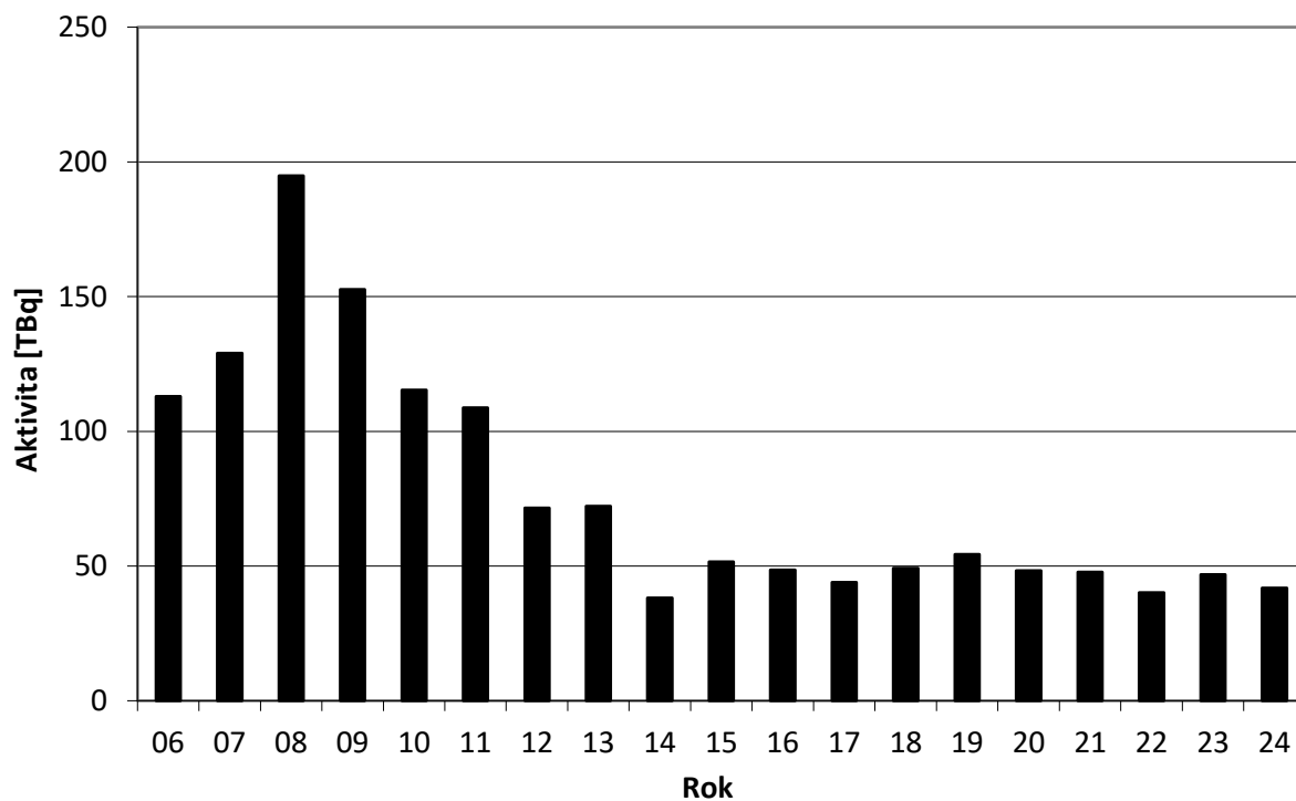
Obr. 15a Bilance plyných výpustí – vzácné plyny ( ^{41}\text{Ar} ) z odběrů ve ventilačním komínu ÚJV Řež v období 2006 – 2024 (vzorkování a měření ÚJV Řež)
