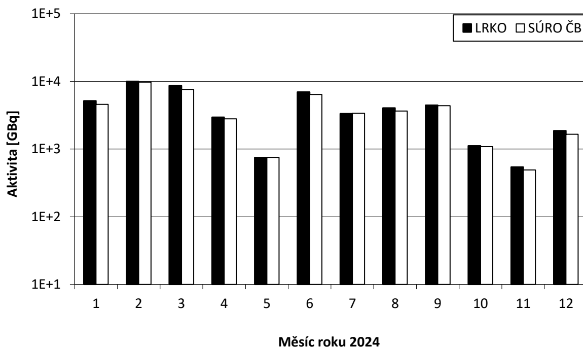
Obr. 20a Celková aktivita ^3\text{H} vypouštěná do vodoteče z JE Temelín v roce 2024 (porovnání hodnot naměřených SÚJB a LRKO provozovatele, odběr JE Temelín, měření SÚRO České Budějovice a LRKO JE Temelín)
