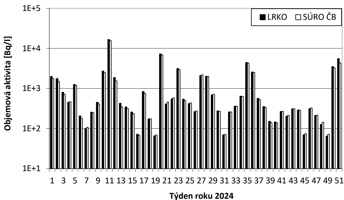
Obr. 19b Objemová aktivita ^3\text{H} v odpadním kanále JE Dukovany v roce 2024 (porovnání hodnot naměřených SÚRO a LRKO provozovatele, odběr JE Dukovany, měření SÚRO České Budějovice a LRKO JE Dukovany)
