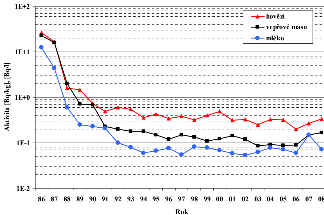
Obr. 13a Průměrné roční hmotnostní aktivity ^{137}\text{Cs} ve vepřovém a hovězím maso a objemové aktivity ^{137}\text{Cs} v mléce od roku 1986 (vzorkování a měření SÚJB RC a SÚRO)
