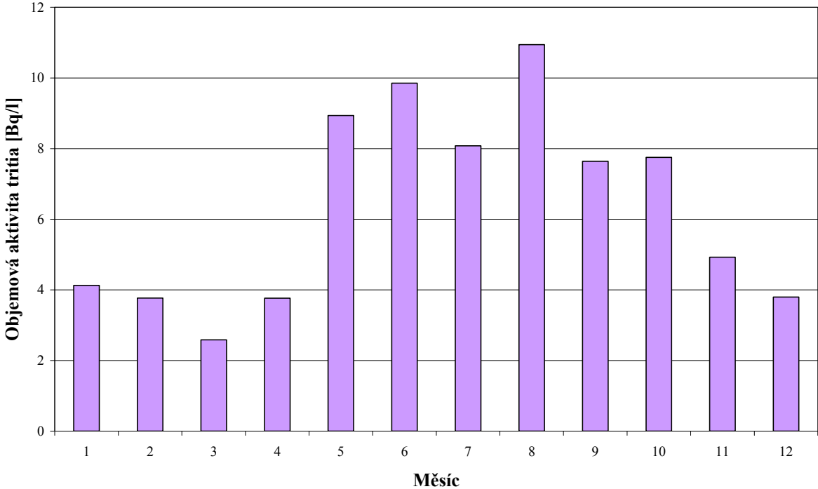
Obr. 12a Objemová aktivita ^3\text{H} v povrchové vodě v roce 2008 – povodí Labe – profil Hřensko (Labe) (vzorkování a měření Povodí, s.p., VÚV TGM Praha)
